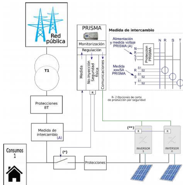
Figura 2 Esquema unifilar
