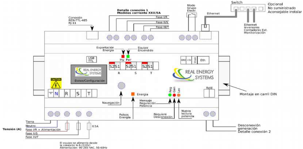
Figura 2 Esquema unifilar
